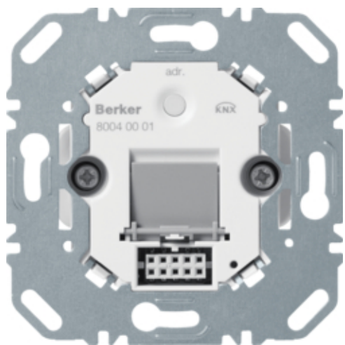
Bus coupling unit flush-mtd, ext. temp. sensor, KNX
