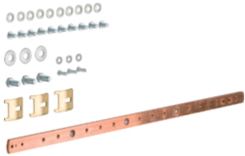
PE busbar, univers, Cu 20 x 5 mm, 2fields
